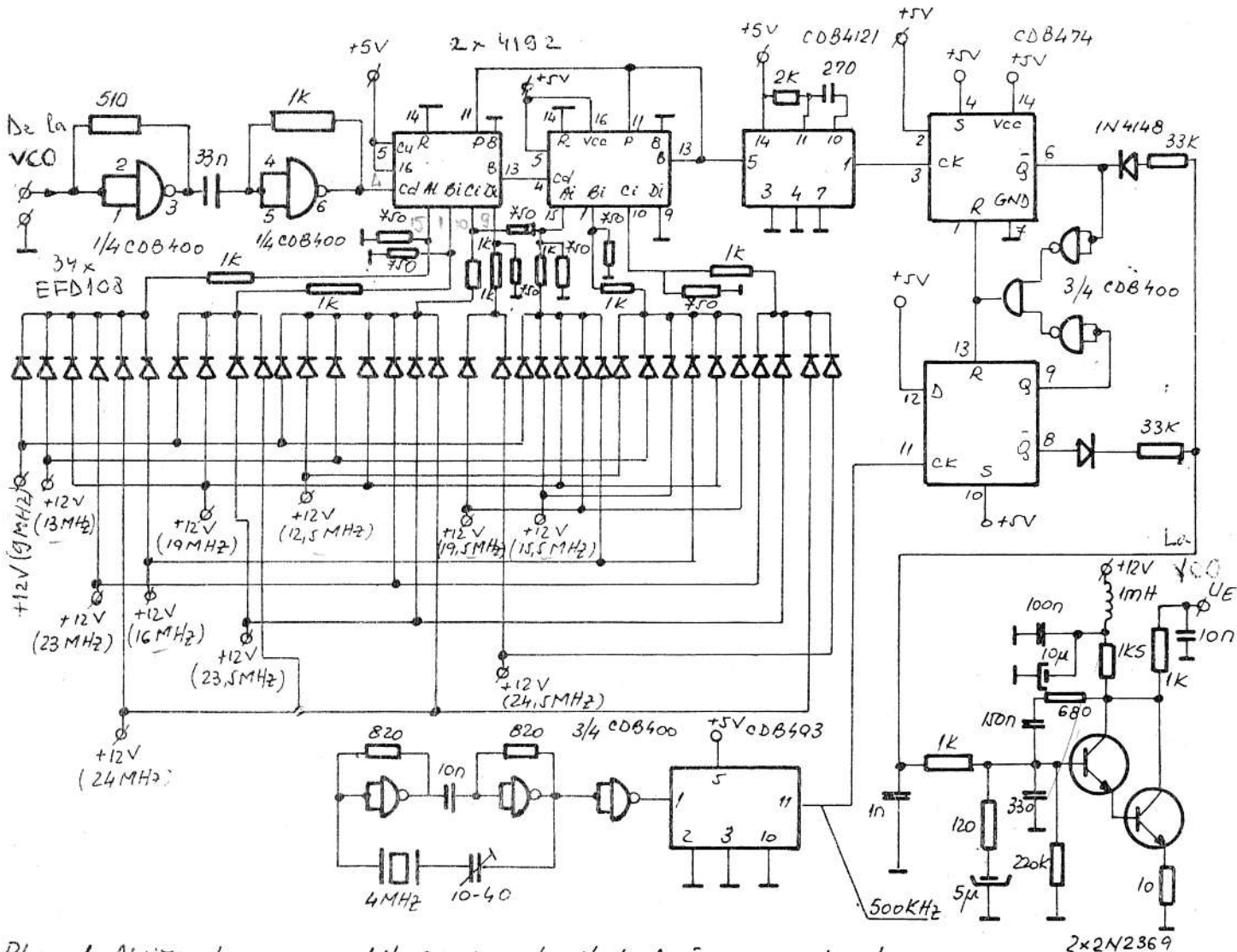
Placa 1: Divizorul programabil, comparatorul de fază, generatorul frecvenței de referință.
