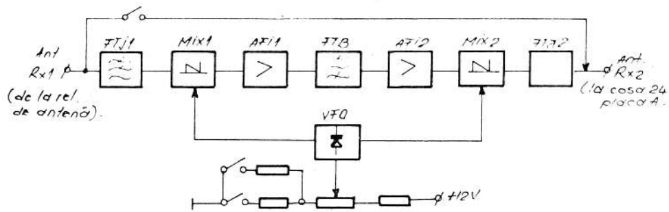
Fig. 1. Convertor medie frecvență.
