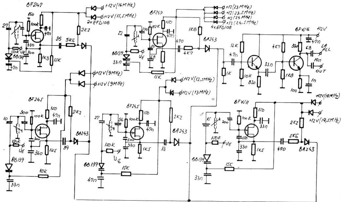
Placa 2: Oscilatoarele comandate în tensiune
